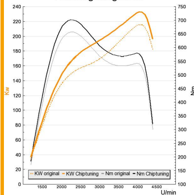
Leistungsdiagramm
